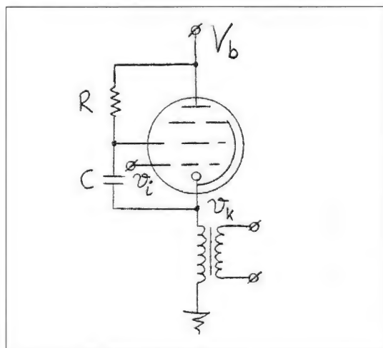
fig.30 Penthode als kathodevolger.
